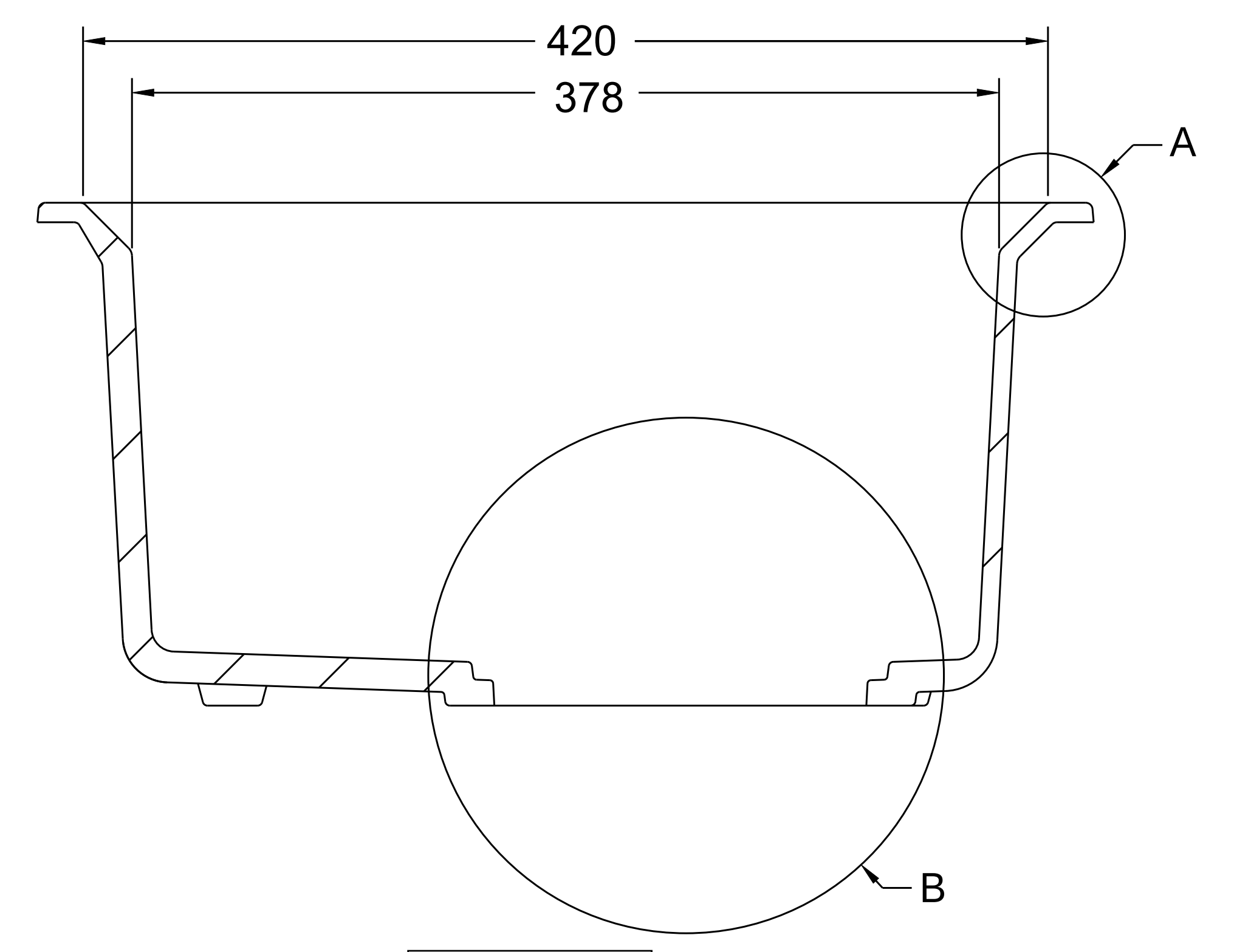
断面 A-A
